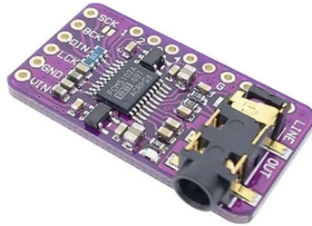
Figura 4: Módulo basado en PCM5102
