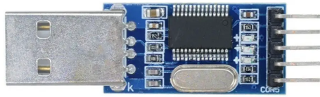
Figura 8: Adaptador basado en PL2303
