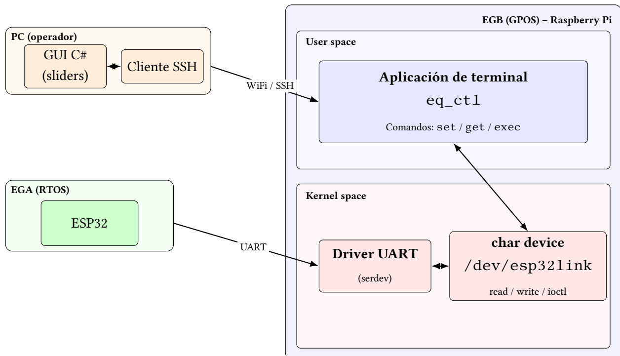
Figura 13: Diagrama de software integrado EGA+EGB.
