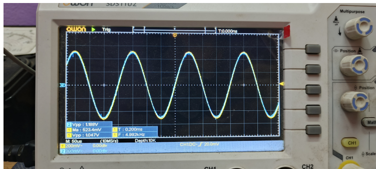
Figura 19: Captura de osciloscopio para senoidal de 5 kHz sin modificar
