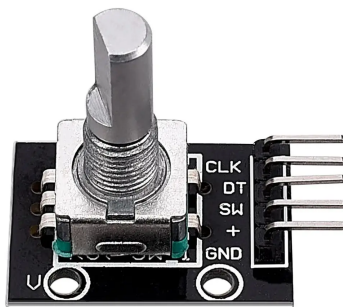
Figura 7: Encoder rotativo KY-040
