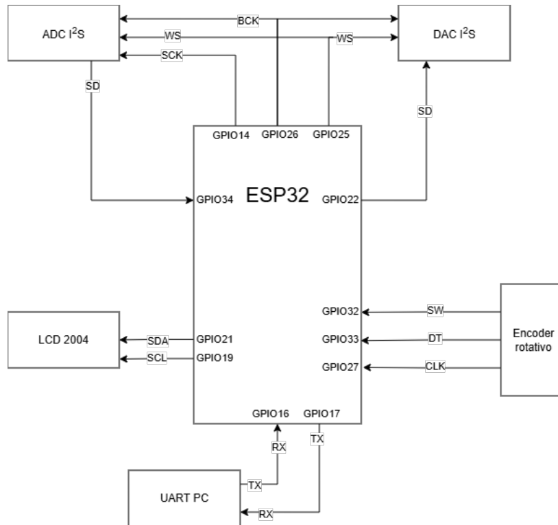
Figura 1: Diagrama en bloques del sistema integrado.
