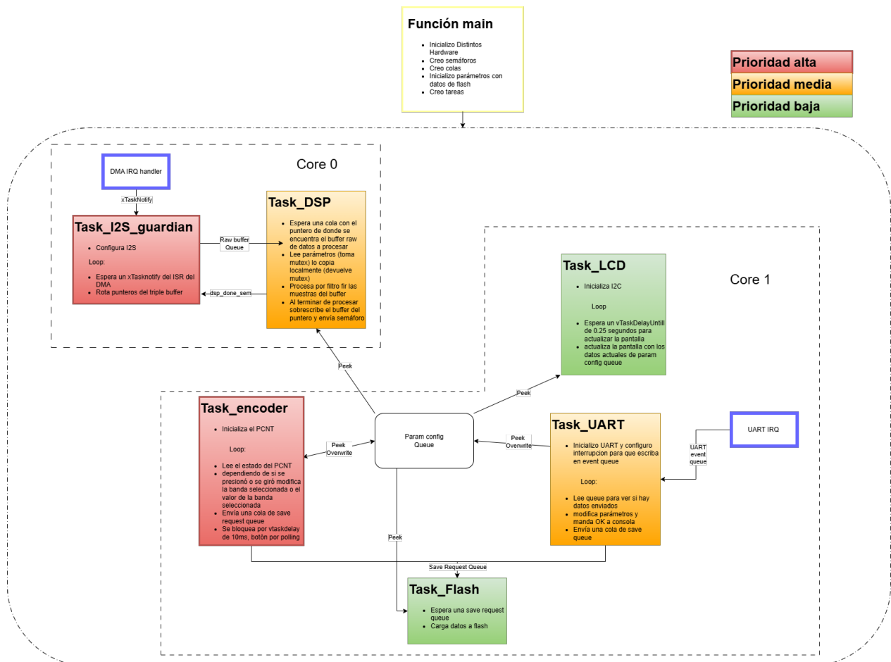
Figura 12: Diagrama de tareas del RTOS actualizado (incluye Task_UART para GPOS)
