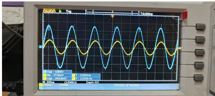
Figura 18: Captura de osciloscopio para senoidal de 2 kHz con atenuación de 10 dB
