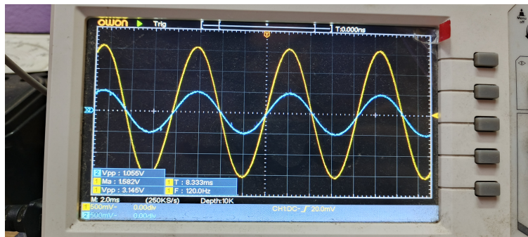
Figura 17: Captura de osciloscopio para senoidal de 120 Hz con ganancia de 10 dB
